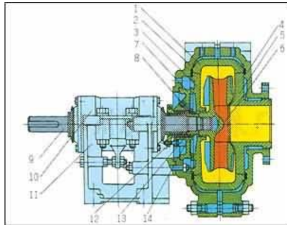
1. 涡壳 2. 泵体 3. 护板 4. 泵盖 5. 前护板 6. 叶轮 7. 填料箱 8. 轴套 9. 泵轴 10. 轴承体 11. 托架 12. 对开填料压盖 13. 填料 14. 水封环
